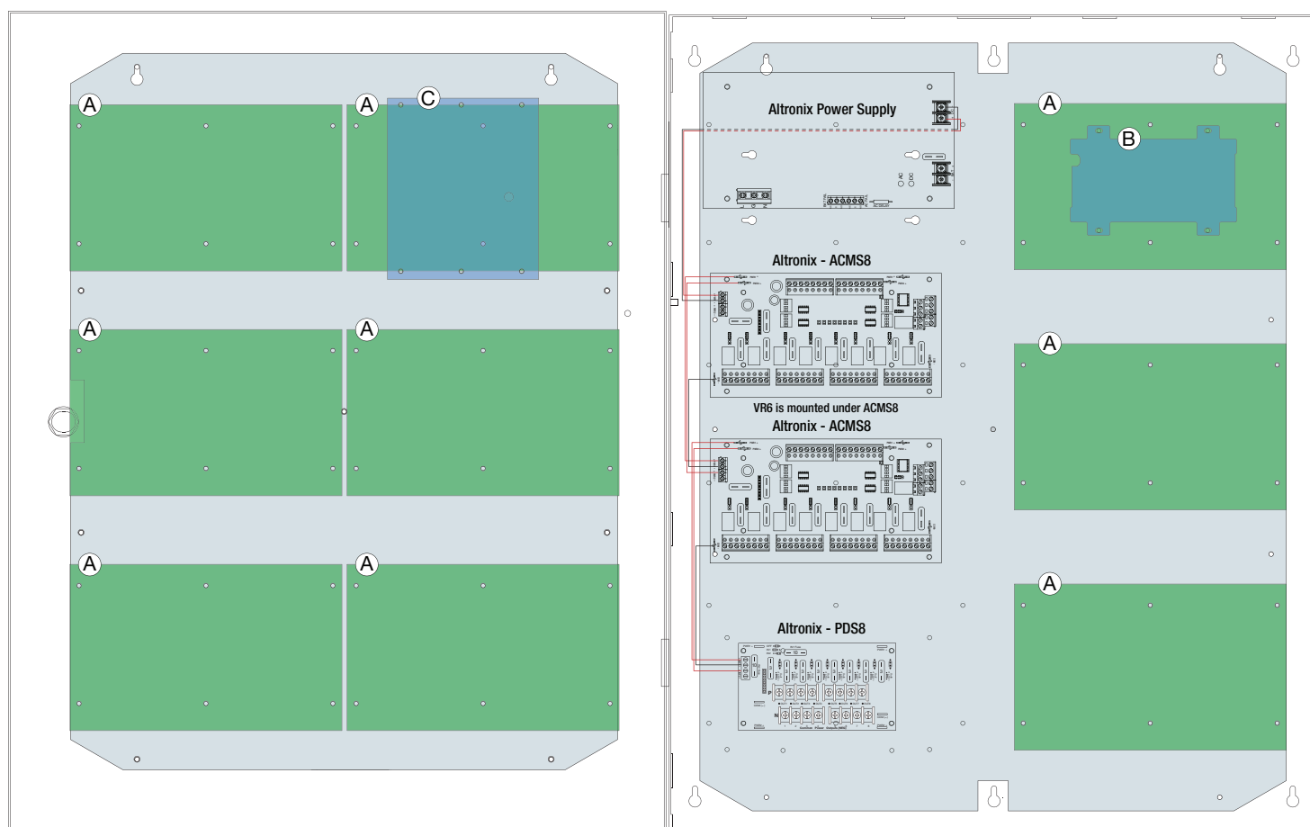
THWD2 Door Backplane
