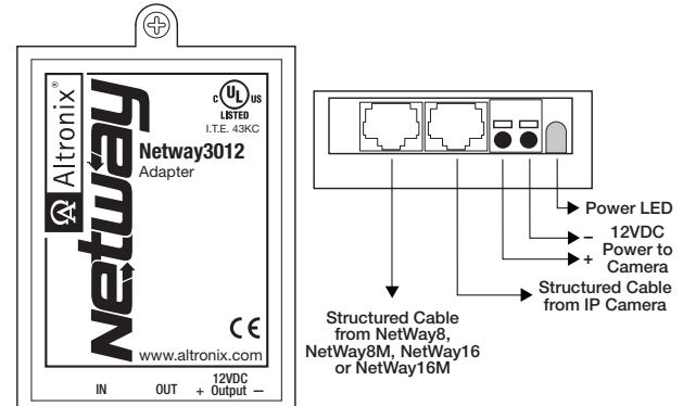
Fig. 3 - NetWay3012
