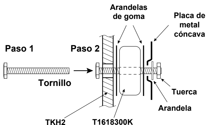
Fig. 1 - Montaje de T1618300K en un backplane
