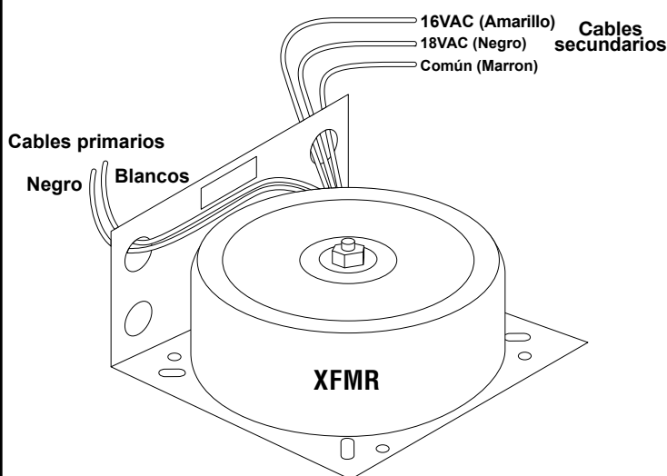
Fig. 2 - Configuración del cableado:
