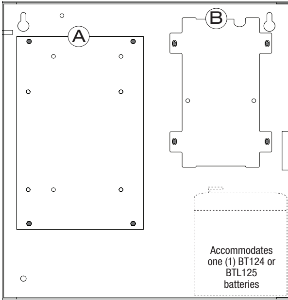
Fig. 2 - TM250 Configurations
