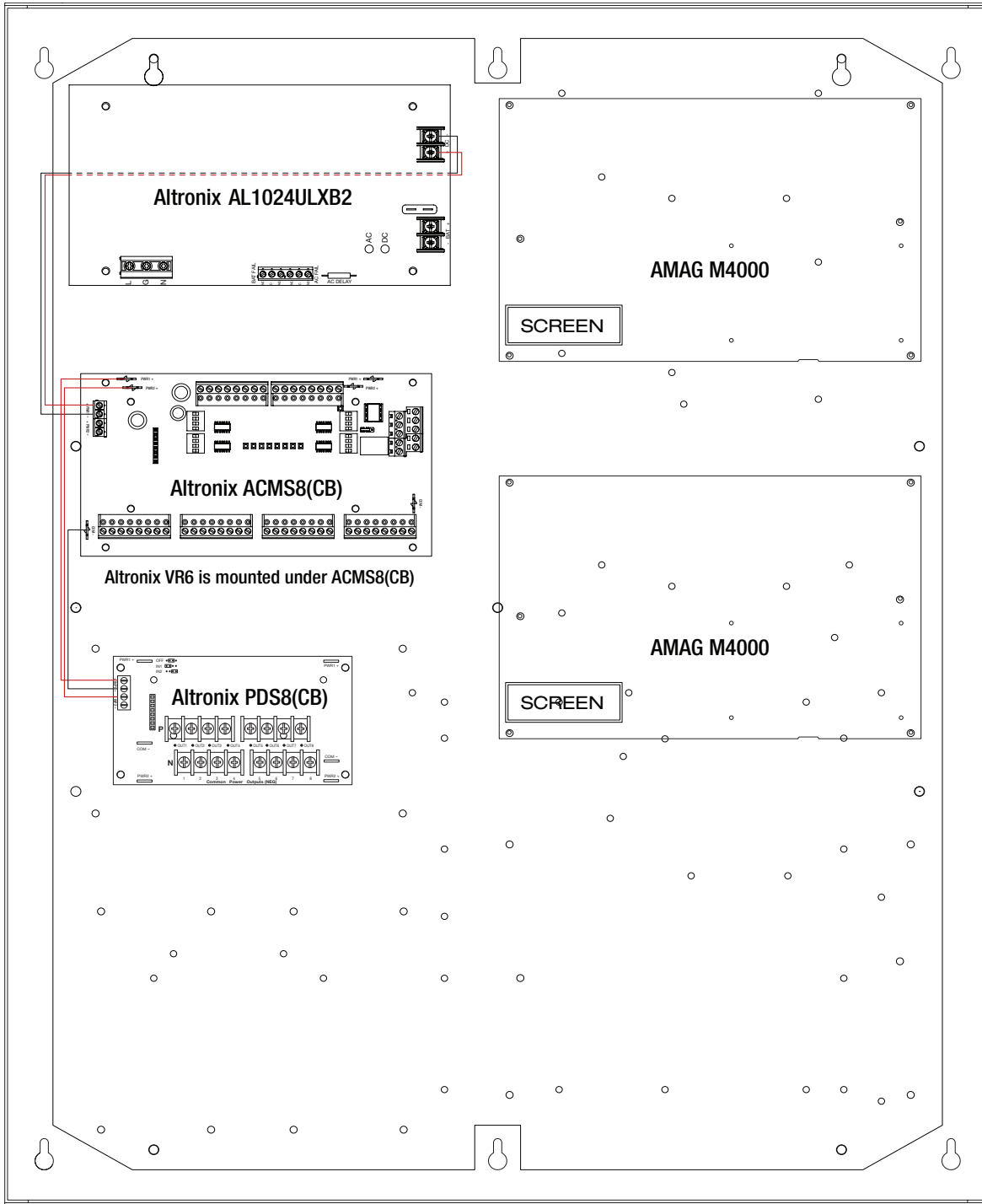
Fig. 3 - T2AGK78S(D) Configuration
