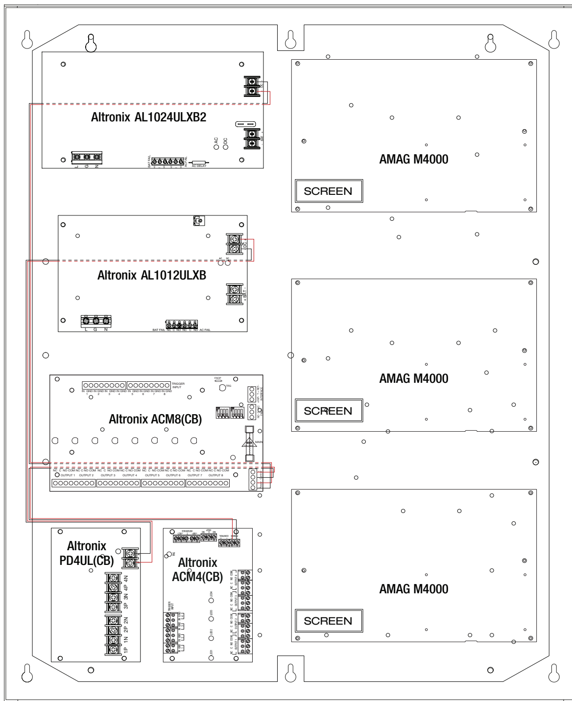
Fig. 6 - T2AGK7512(D) Configuration
