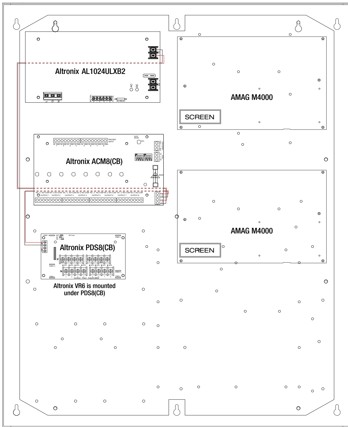
Fig. 2 - T2AGK78(D) Configuration
