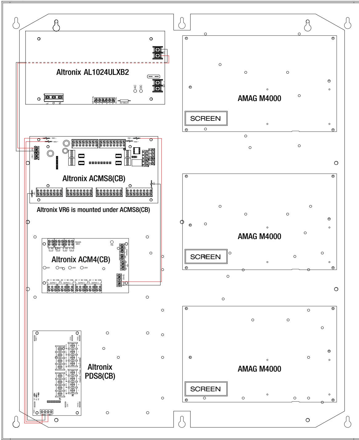
Fig. 5 - T2AGK712S(D) Configuration
